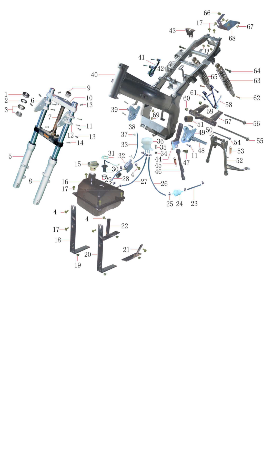
图1 铁件部分
